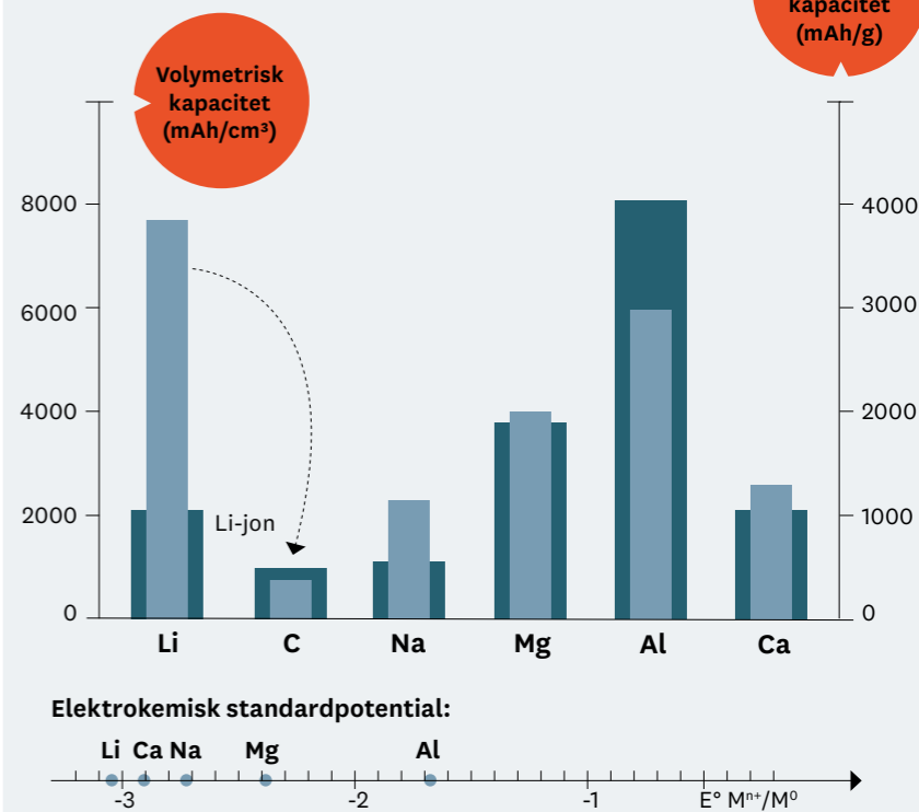
Diagrammet visar kapacitet för olika negativa elektrodmaterial. Den streckade pilen visar hur kapaciteten minskar när man går från metalliskt litium till litium interkalerat i grafit (C) som i litiumjonbatteriet.
